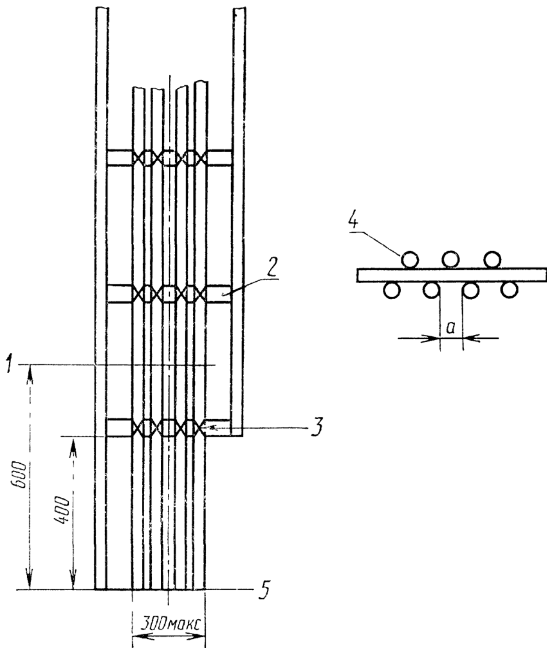
1—центральная линия горелки; 2—круглые стальные перекладины; 3—стальные проволочные крепления; 4—способ расположения кабелей на обеих сторонах лестницы; 5—пол; a —расстояние между закрепленными образцами Черт. 5
