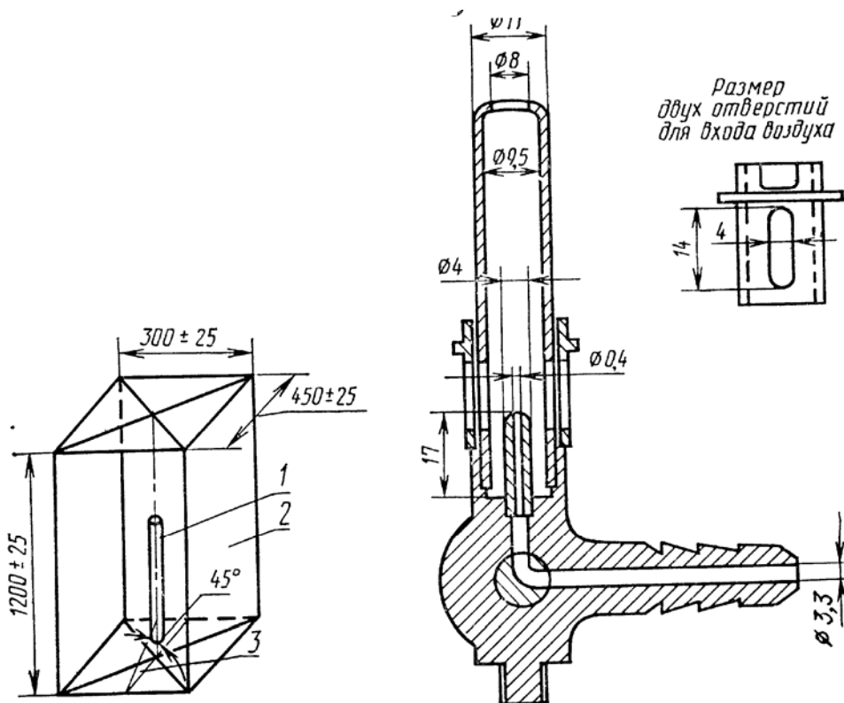
1—образец кабеля; 2—испытательная камера; 3—ось горелки Черт. 1
