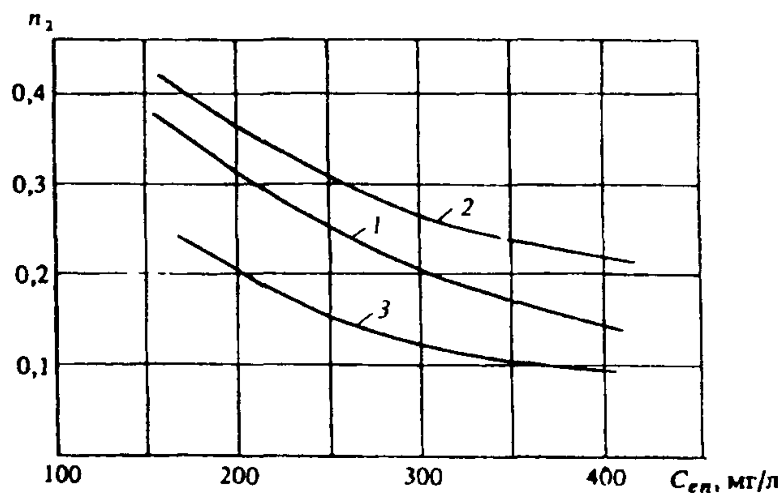
Черт. 2. Зависимость показателя степени n_2 от исходной концентрации взвешенных веществ в городских сточных водах при эффекте отстаивания 1 — \vartheta = 50\% , 2 — \vartheta = 60\% ; 3 — \vartheta = 70\%
